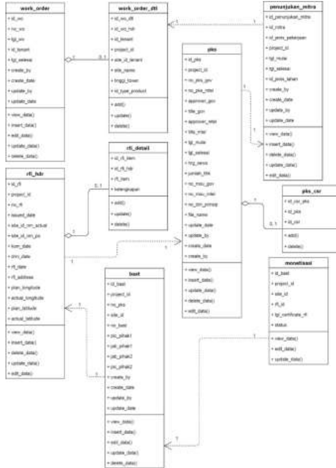
Gambar 4. Class Diagram Sistem Informasi Monitoring Perjanjian Kerja Sama
