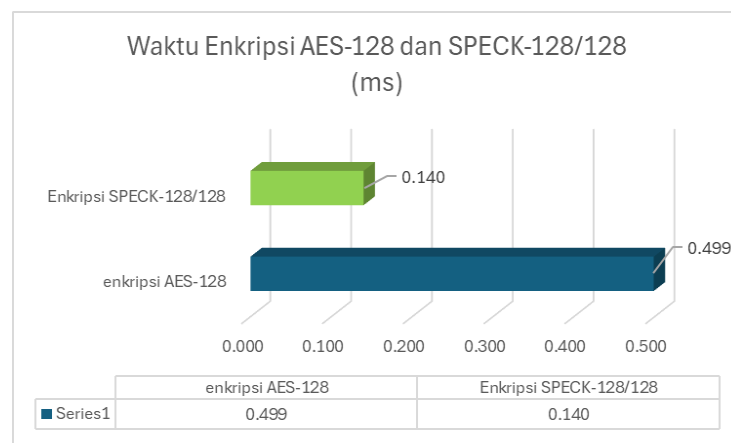
Gambar 11. Waktu Enkripsi AES-128 dan SPECK-128/128
