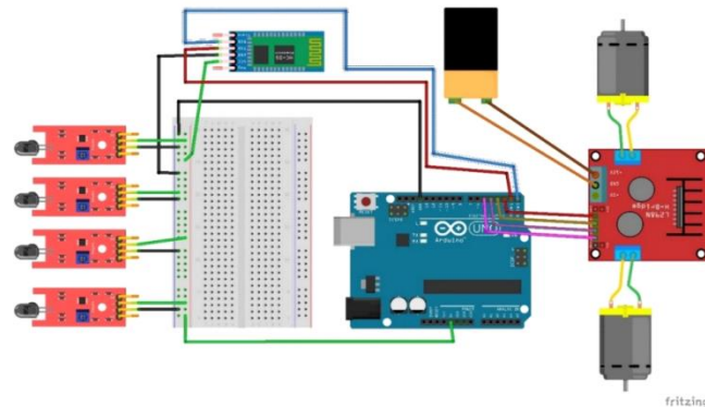
Gambar 3. Desain Alat
